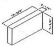
2 1/4 x 8 x 16
